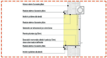
PARTICOLARE FINESTRA E INBOCCE SCALA 1:20
