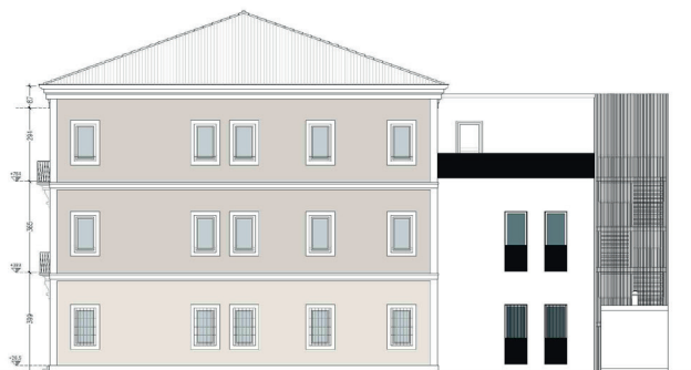
Prospetto EST
