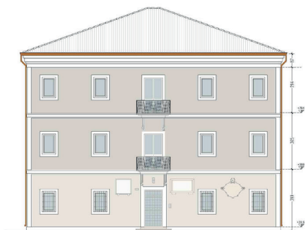
Prospetto SUD
