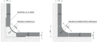
PARTICOLARI SGUSCIA PAVIMENTO-RIVESTIMENTO IN PIASTRELLE DI GRES SC. 1:1 (POSA ALTERNATIVA SGUSCIA METALLICA O SGUSCIA IN GRES PEZZO SPECIALE)
