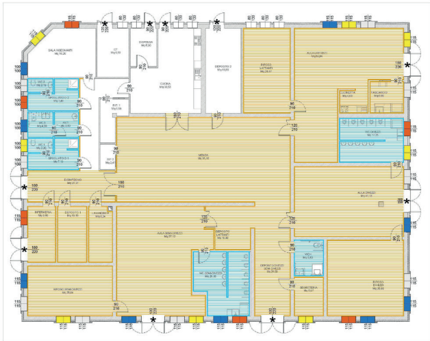
PANTA PIANO TERRA SCALA 1:100 BATTISCOPA-SGUSCIA DI RACCORDO PAVIMENTO-RIVESTIMENTO
